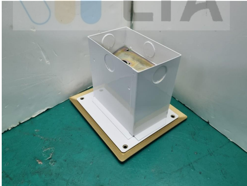
<측면 사진>
